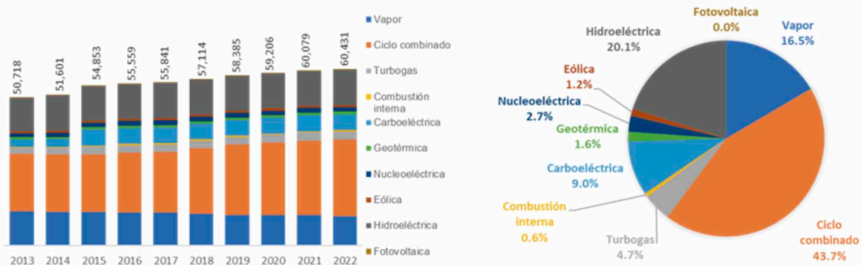
Izq. Capacidad instalada de generación eléctrica por tipo de tecnología 2013 a 2022 (Megawatts)/ Der. Contribución a la capacidad instalada por tipo de tecnología 2022 (porcentaje)
