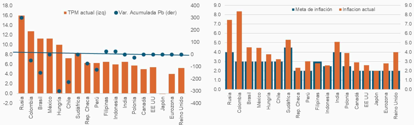
Izq. Tasa de política monetaria (TPM) actual y variación acumulada en puntos base de la TPM en el 4T de 2023 / Der. Diferencia entre la meta inflacionaria y su brecha actual al cuarto trimestre 2023, por países.
